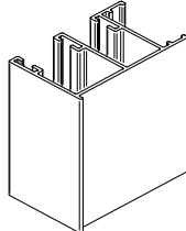
Az "iker" redőnysín 27 x 45 mm
